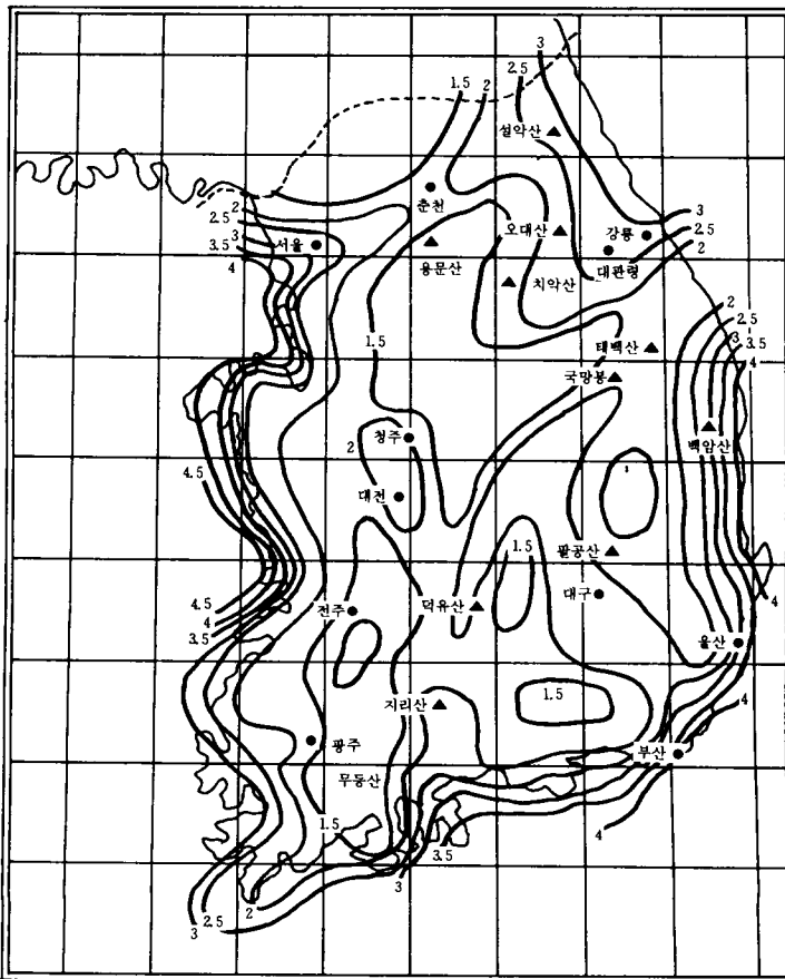
〈그림3〉 봄의 풍속분포도
