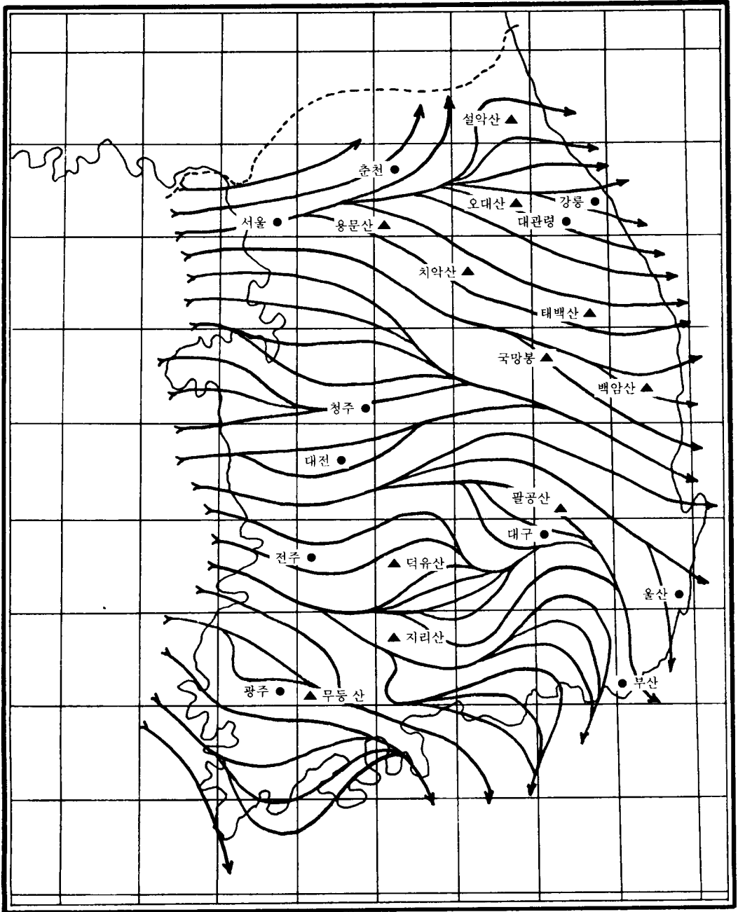
(그림4) 봄의 평균유선도
