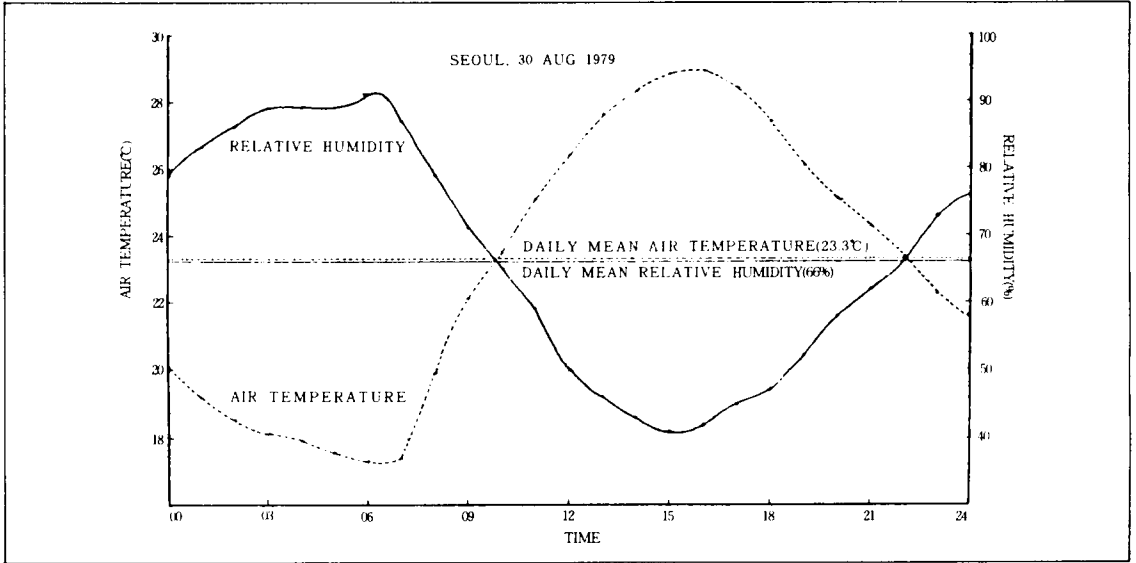
(그림2) 기온과 상대습도의 일변화
