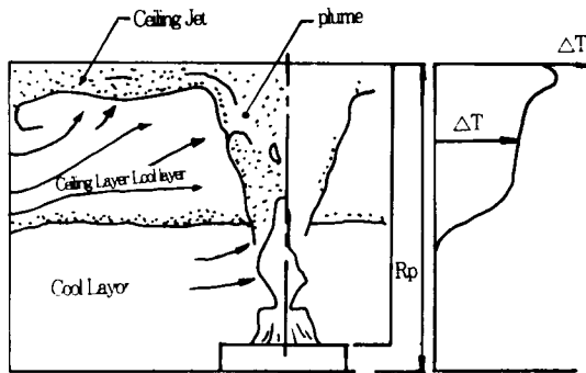
그림 2 室内火災의 Ceiling Layer Flow
