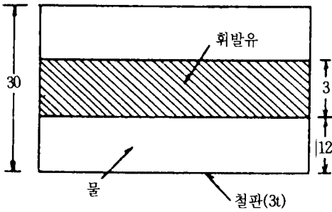
단면도
