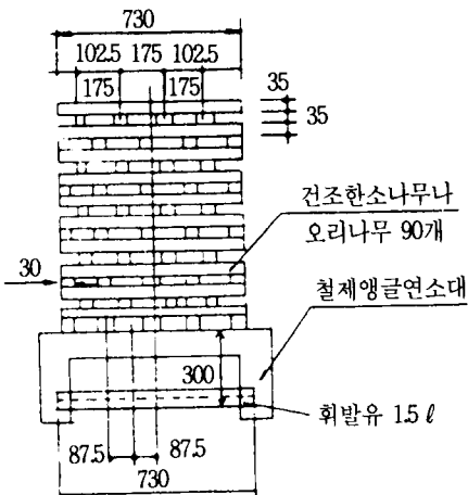
〈정 면 도〉
