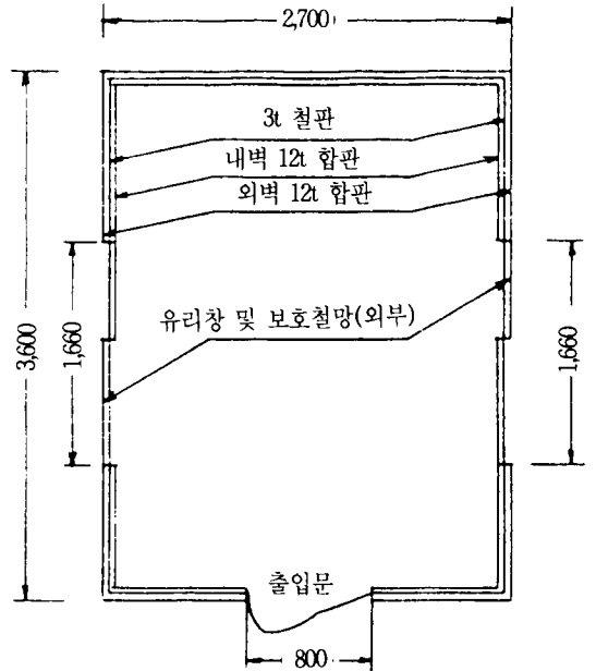
〈평 면 도〉
