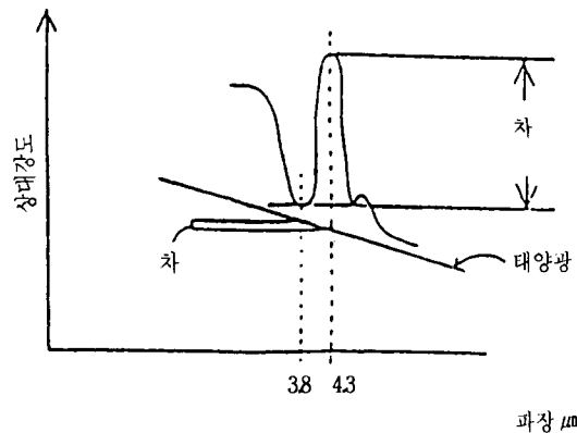
그림 11. 태양광과 불꽃이 공존시의 방사량 차이
