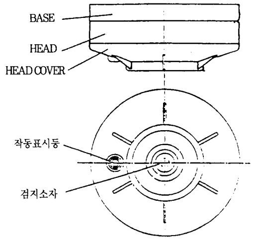
그림3 화염감지기의 외형
