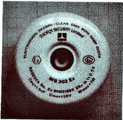
화염 (IR) 감지기 전면 (SAPPHIRE WINDOW, PHOTO SENSOR)
