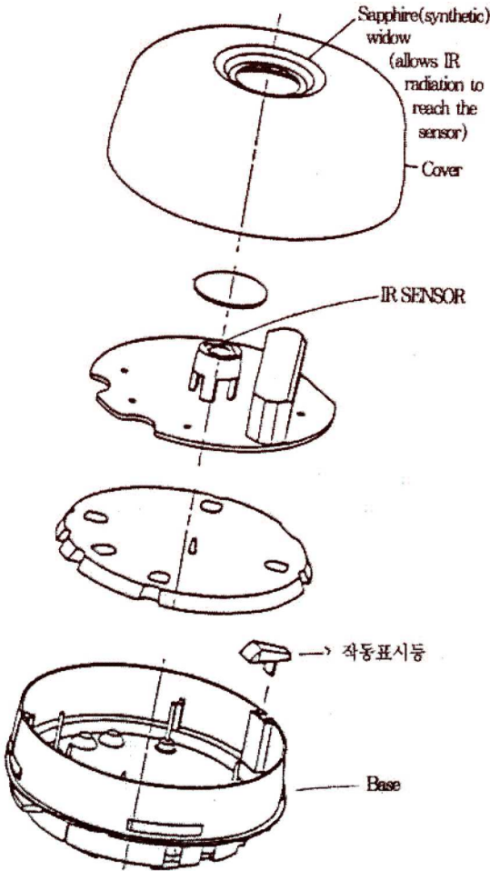
그림 1. IR Flame detector의 구조
