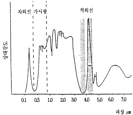
그림 9 가솔린의 연소와 방사파장
