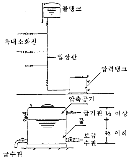
압력수조방식 계통도(例)
