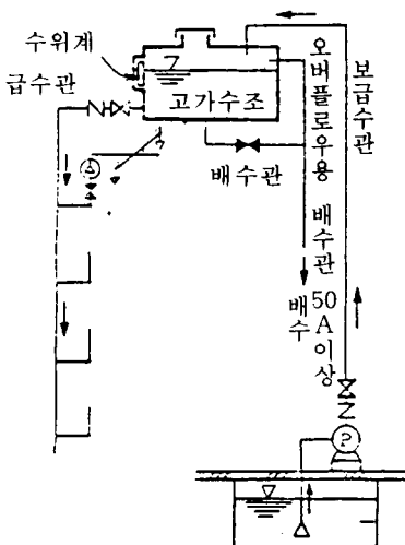
고가수조방식 계통도(例)
