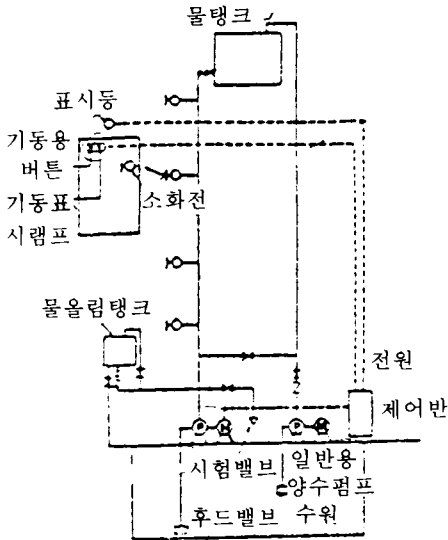
펌프방식 계통도(例)
