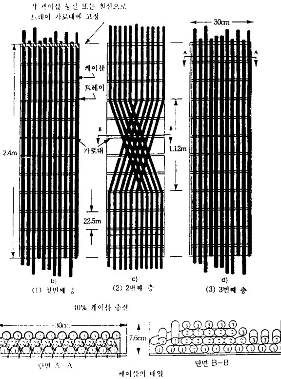
[그림 1] 케이블 트레이 시험체
