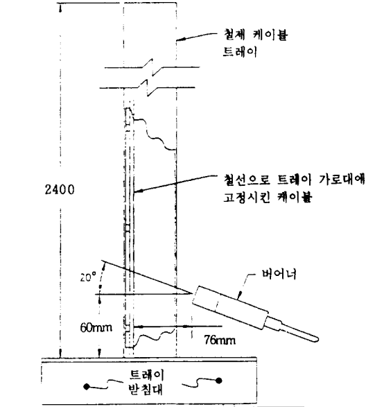
[그림 5] 버어너 설치 위치
