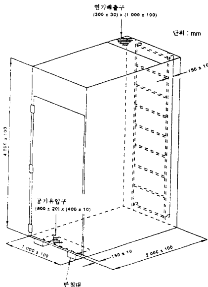
[그림 2] 시험챔버
