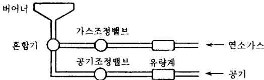
[그림 4] 연소원의 배관 배열
