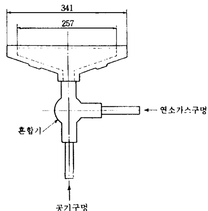
[그림 3] 버어너의 구조 및 크기
