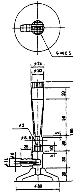
[그림 6] 맥켈버너(단위 : mm)
