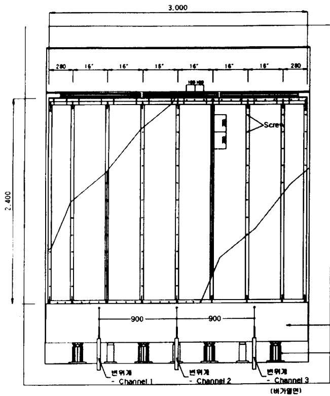
입면도
