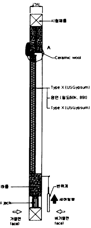
수직단면도
