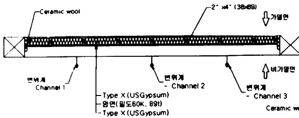
수평단면도
