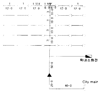
[그림 1] 설계면적의 헤드배치
