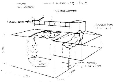
그림1. 샌드위치패널 화재시험장치 개요도
