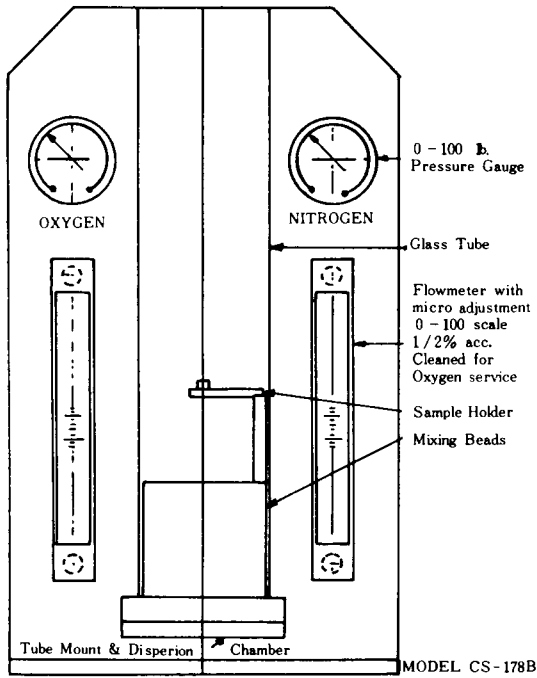
그림 1. 구조도
