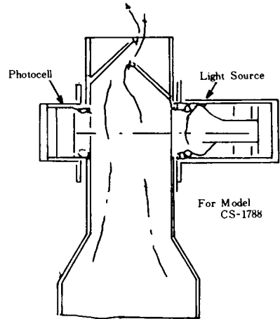
그림 2. 연농도 측정기
