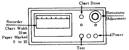
그림 3. 기록계
