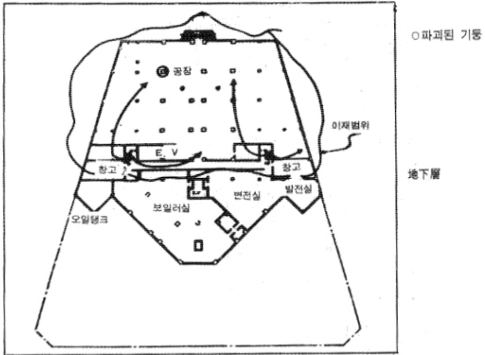
罹災建物 平面圖 (火災狀況 圖示)
