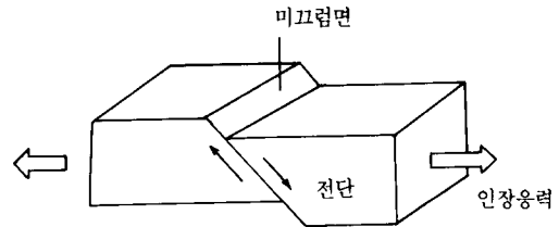
【그림 3】 원자간의 미끄럼면
