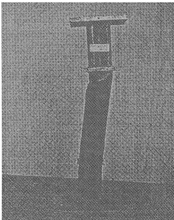
【사진 7】 내화강 각형 강관의 고온시 보, 기둥 시험
