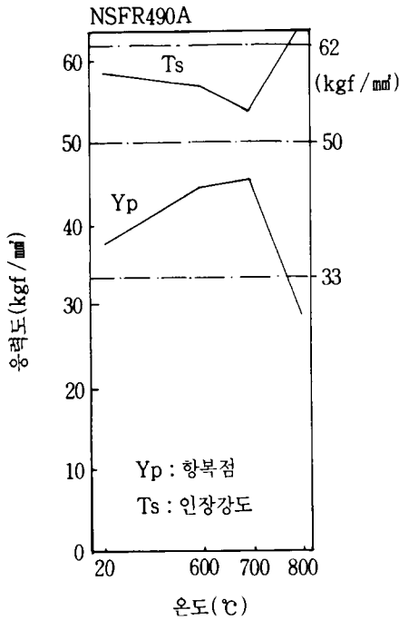
【그림 7】 내화강의 가열 후 강도
