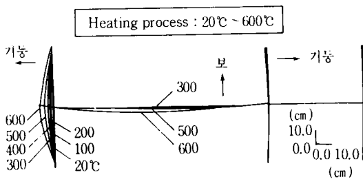
【그림 5】 架構의 열변형(昇溫時)
