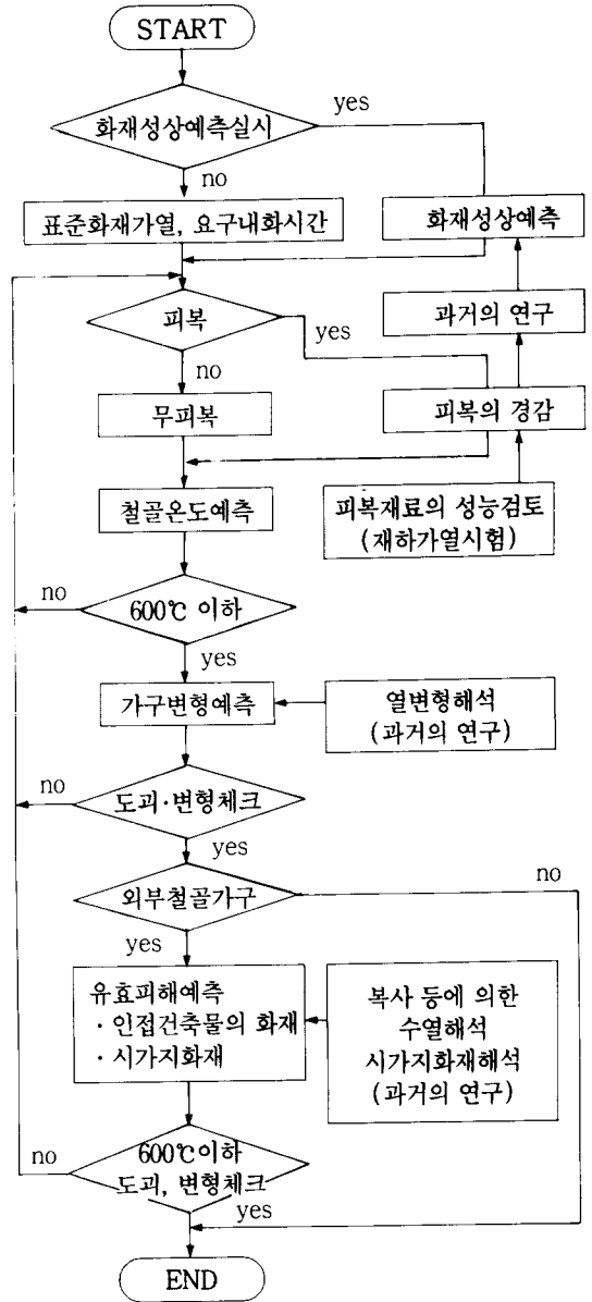
【그림 4】 내화강을 이용한 건물의 내화설계 Flow
