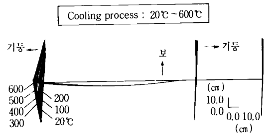
【그림 6】 架構의 열변형(冷却時)
