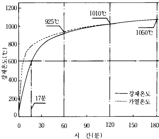
【그림 1】 표준가열곡선과 무피복 철골의 온도상승
