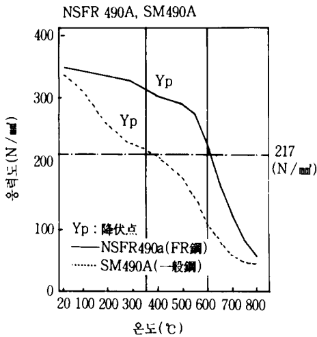
【그림 2】 강재의 고온강도
