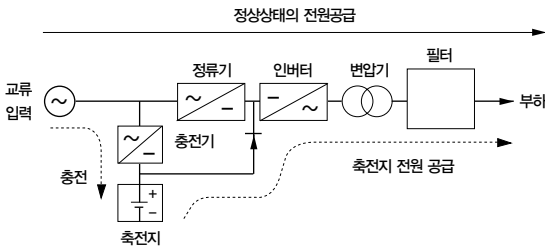
● 그림 2 ● ON-LINE TYPE
