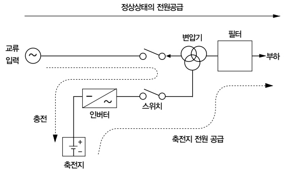
• 그림 4 • LINE INTERACTIVE TYPE
