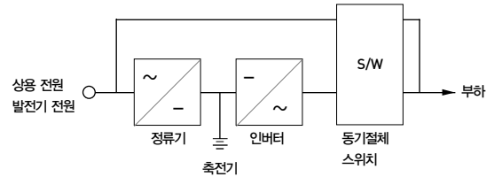
• 그림 1 • UPS의 기본 구성도
