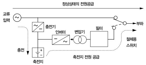
● 그림 3 ● OFF-LINE TYPE
