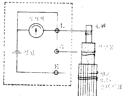
<그림 1> 케이블의 절연저항 측정
