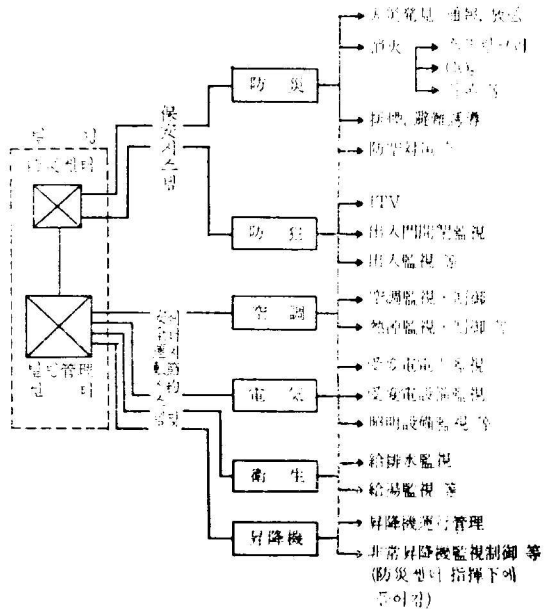
그림 (2) 빌딩 設備制御의 시스템의 關係
