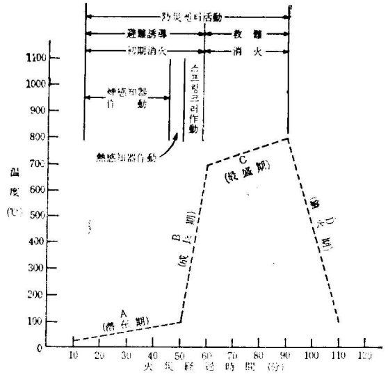
그림 (3) 火災經過時間과 溫度分布類型 모델 및 各 設備와의 關係
