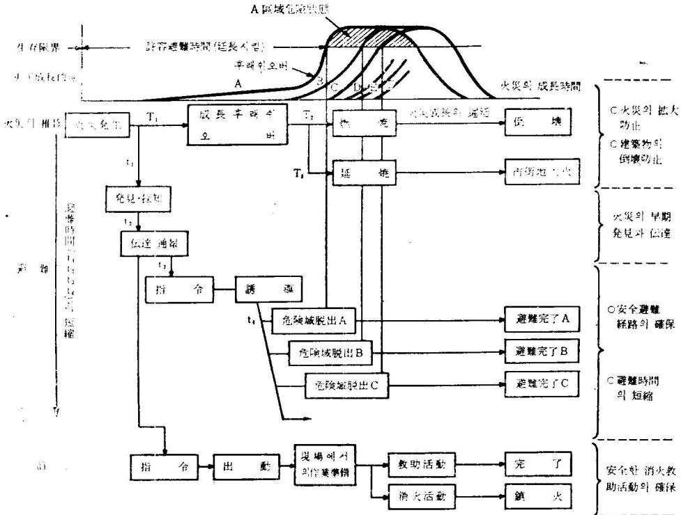
그림 (4) 建築群에 대한 防災計劃
