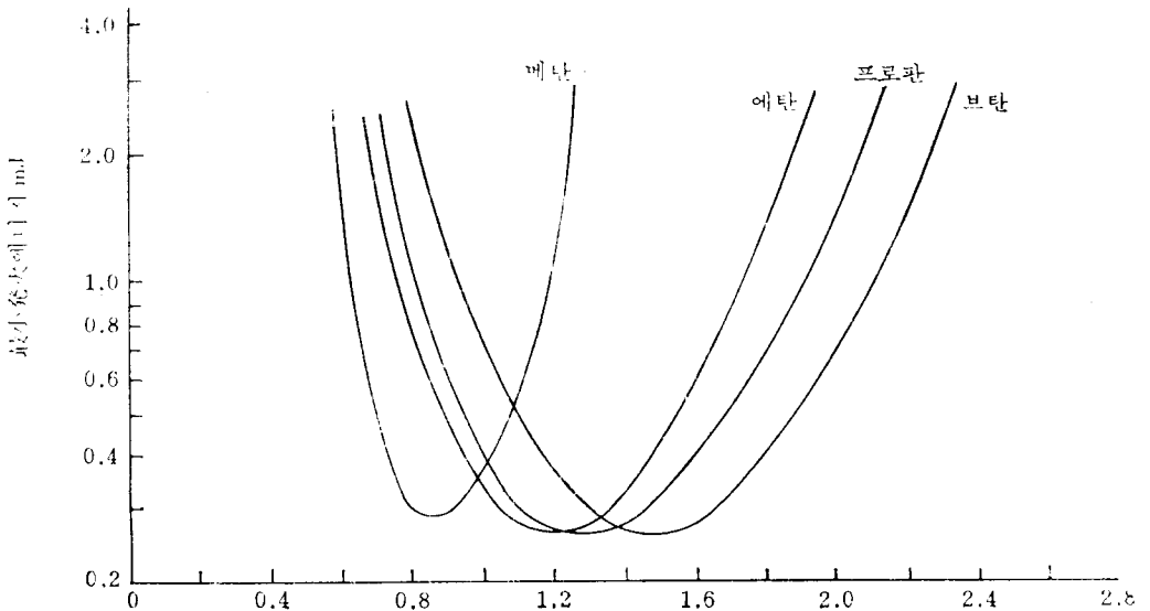
그림 (3) 空氣와의 混合가스의 最小發火에너지
