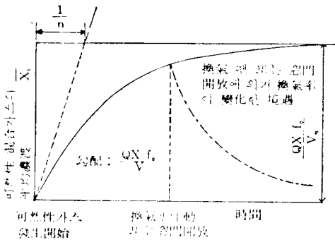
그림 (2) 可燃性 混合가스의 平均濃도와 時間變化
