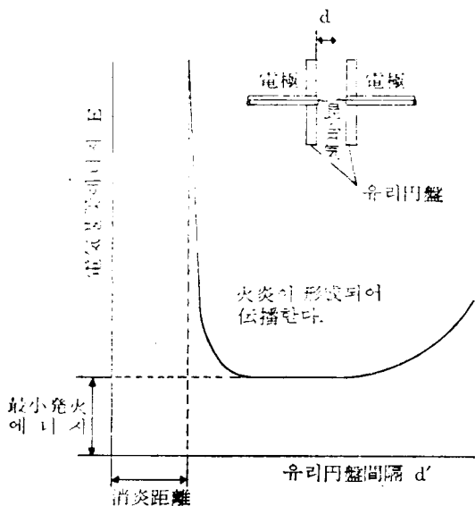
그림 (4) 最小發火에너지와 消炎距離의測定
