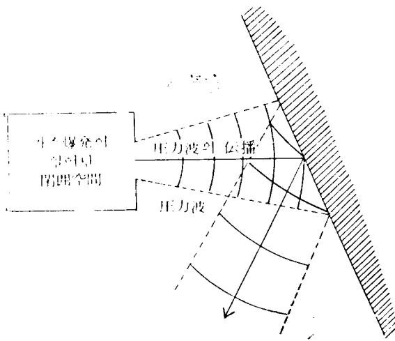
그림 (7) 壓力波의 傳播
