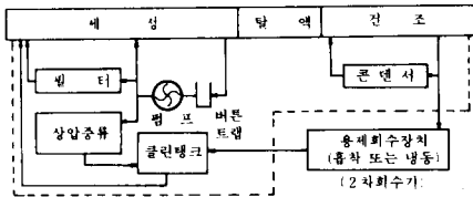
〈도표 1-3〉 세정·탈액·건조겸용기 (hot machine) (증류있는 경우)
