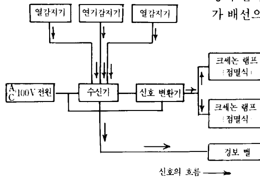
◀그림 2. 신체장애자 시설용 화재 경보장치의 구성도.
