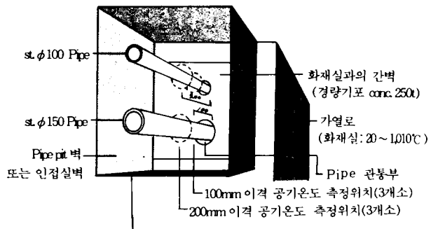
〈그림 1〉 시험체 모형도
