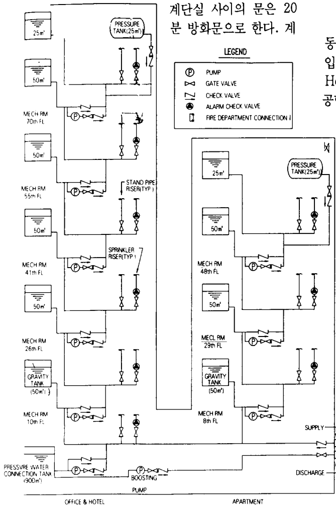
(SPRINKLER & STAND PIPE SCHEMATIC)
