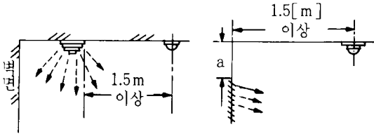
〈그림 3〉 공기 유입구의 감지기 설치
