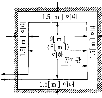
〈그림 6〉 공기관 상호간격
