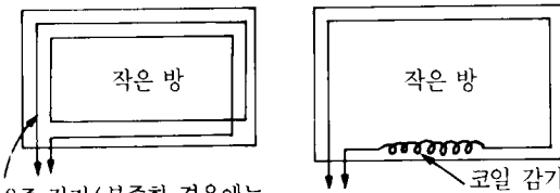
〈그림 5〉 공기관의 노출부분
