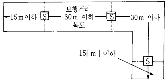
〈그림 9〉 복도 및 통로의 감지기 설치
