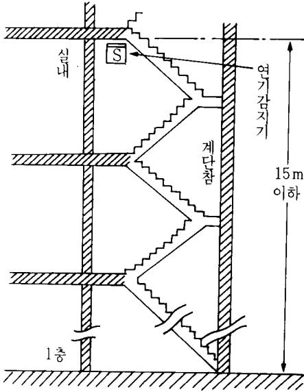
〈그림 10〉 계단 및 경사로의 감지기 설치
