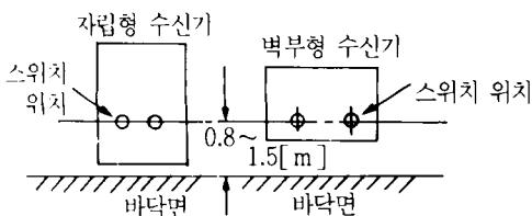
〈그림 11〉 조작부 설치위치
