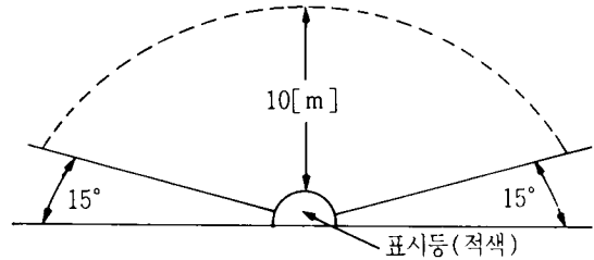
〈그림 14〉 표시등의 식별
