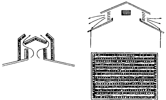
<그림 4> 자연 환기구 형태
