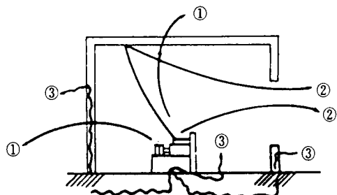
(그림 1) 공장소음 전달 경로계통
