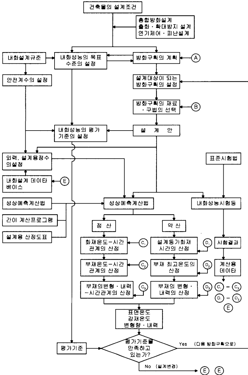
(그림 3) 내화설계의 기본 프레임
